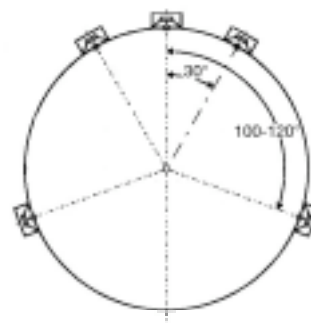
Figure 1. Disposition des haut-parleurs recommandés par la norme ITU-R BS.775.
