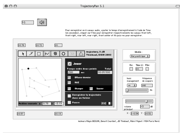
Figure 6. Interface de l'outil de panoramisation 5.1.
