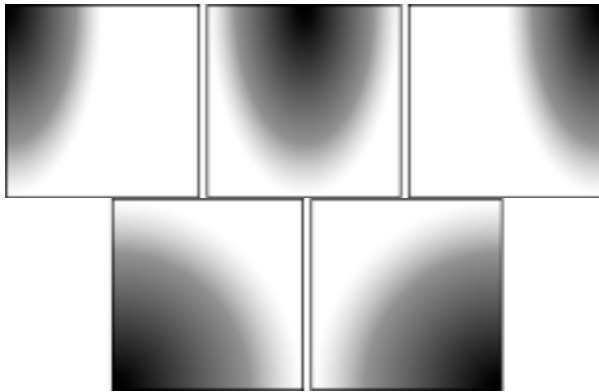
Figure 3. Représentation du gain en fonction de la position de la source virtuelle pour chaque haut-parleur (gauche, centre, droit, surround gauche et surround droit).
