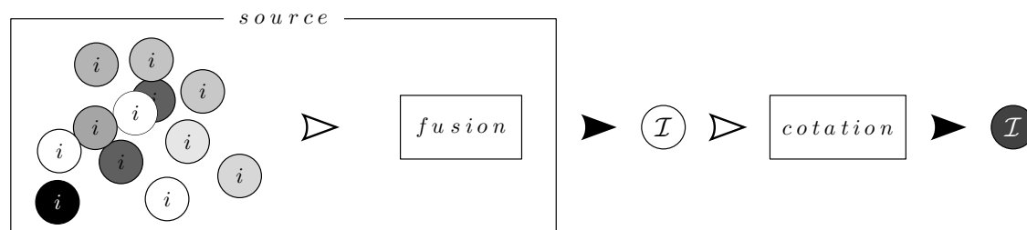
FIGURE 6.3 – Fusion d’informations atomiques et cotation de connaissances
