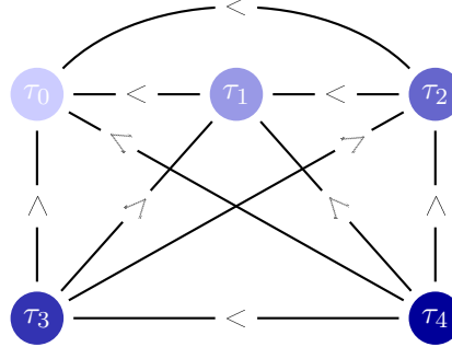
FIGURE 5.1 – Un exemple de treillis de De Morgan : (\mathcal{L}_5, \wedge, \vee, >)
