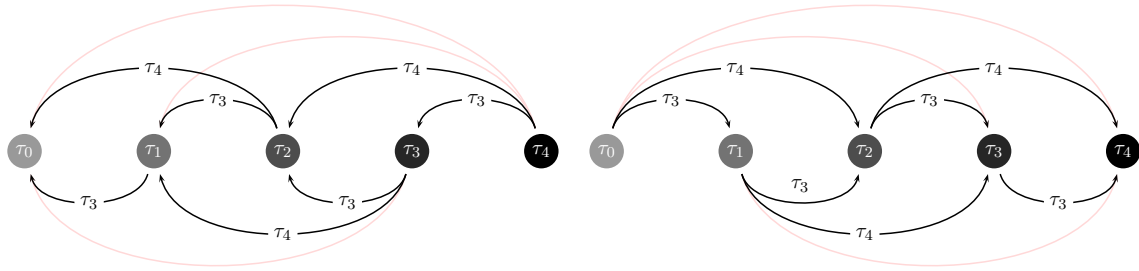
FIGURE 5.8 – Les conditions stratégiques de \tilde{F}_i(\tau_\alpha, \tau_\beta) (à gauche) et de \tilde{F}_c(\tau_\alpha, \tau_\beta) (à droite) pour l'utilisateur 1
