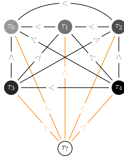
FIGURE 5.4 – Demi-treillis inférieur (\mathcal{L}_5 \cup \{\tau_?\}, \wedge, <)
