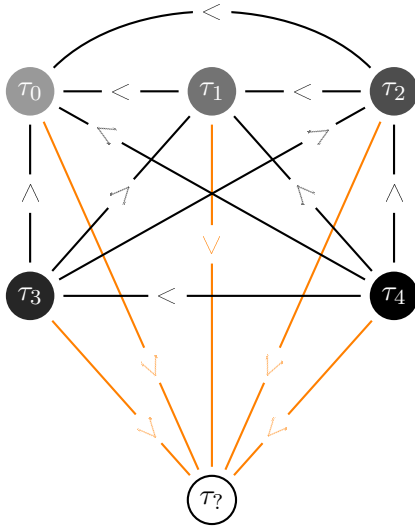
FIGURE 5.3 – Demi-treillis supérieur (\mathcal{L}_5 \cup \{\tau_?\}, \vee, >)
