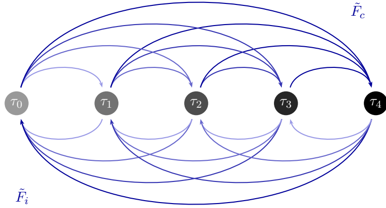
FIGURE 5.7 – Représentation graphique de G(\tau_\alpha, \tau_\beta, \tau_\gamma) , allégée des seuils
