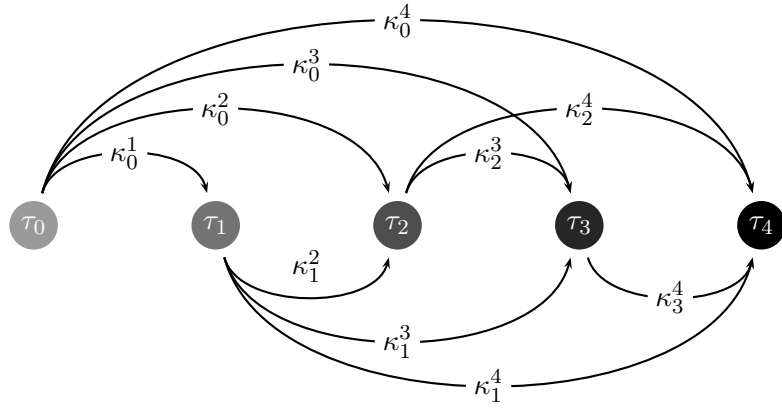
FIGURE 5.6 – Représentation graphique des conditions stratégiques de \tilde{F}_c(\tau_\alpha, \tau_\beta)
