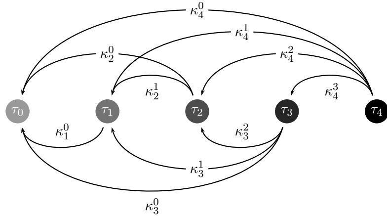
FIGURE 5.5 – Représentation graphique des conditions stratégiques de F(\tau_\alpha, \tau_\beta)
