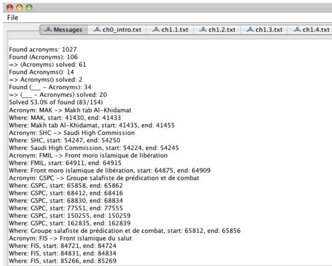
FIGURE 7.5 – Statistiques de la résolution d'acronymes
