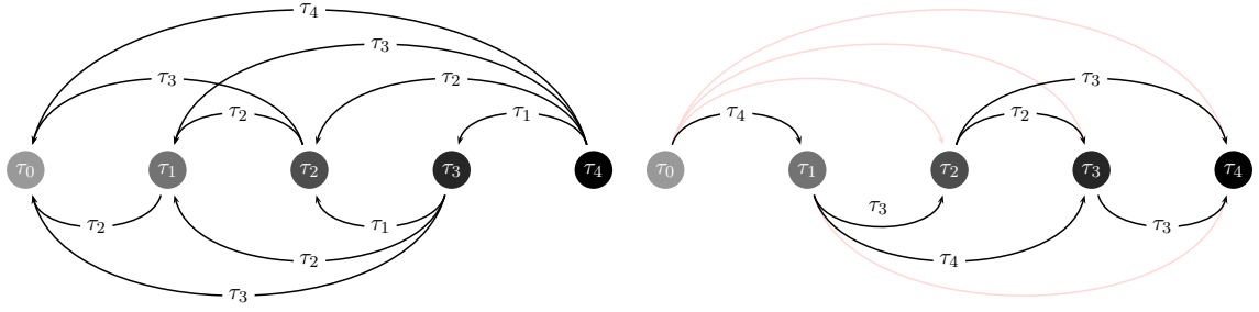
FIGURE 5.9 – Les conditions stratégiques de \tilde{F}_i(\tau_\alpha, \tau_\beta) (à gauche) et de \tilde{F}_c(\tau_\alpha, \tau_\beta) (à droite) pour l'utilisateur 2
