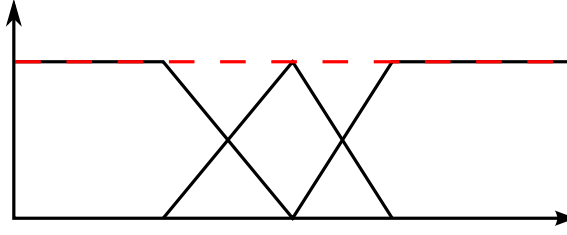
FIGURE 5.2 – Incertitude totale sur une partition floue (en pointillés )
